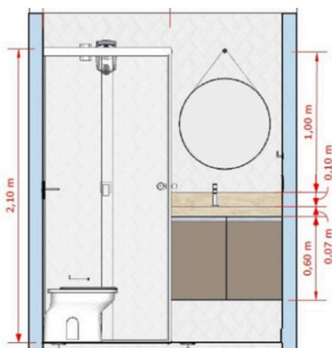
VISTA FRONTAL ESCALA 1:20
